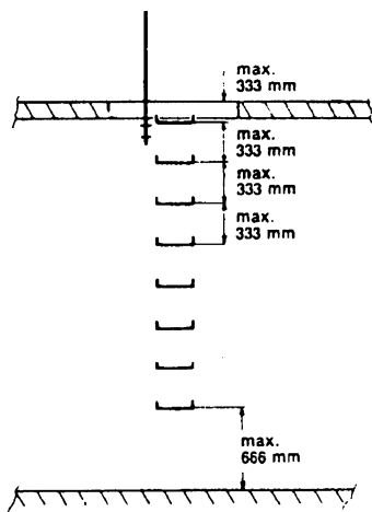
Bild 4: Einläufiger Steigeisengang
